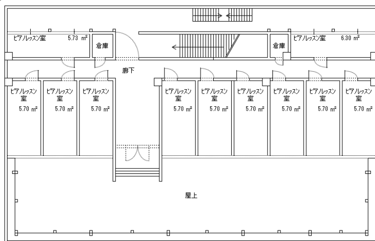
5 階 平 面 図
